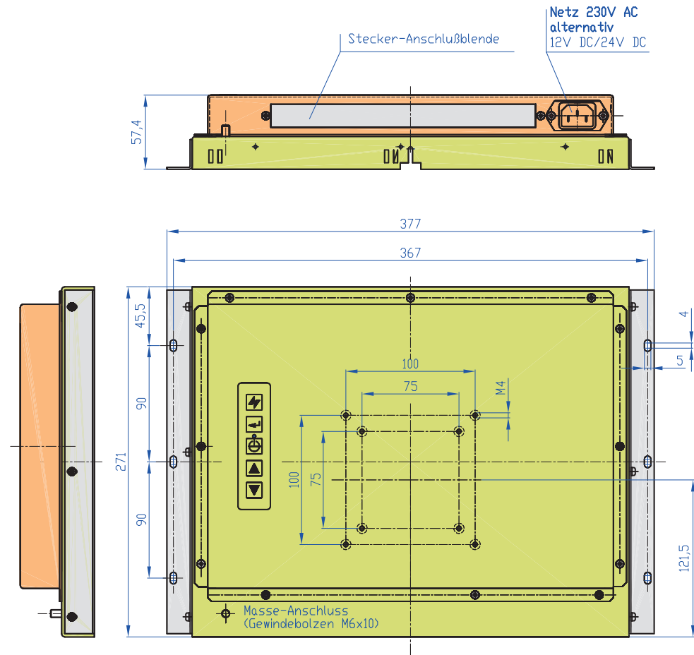
RÜCKANSICHT
