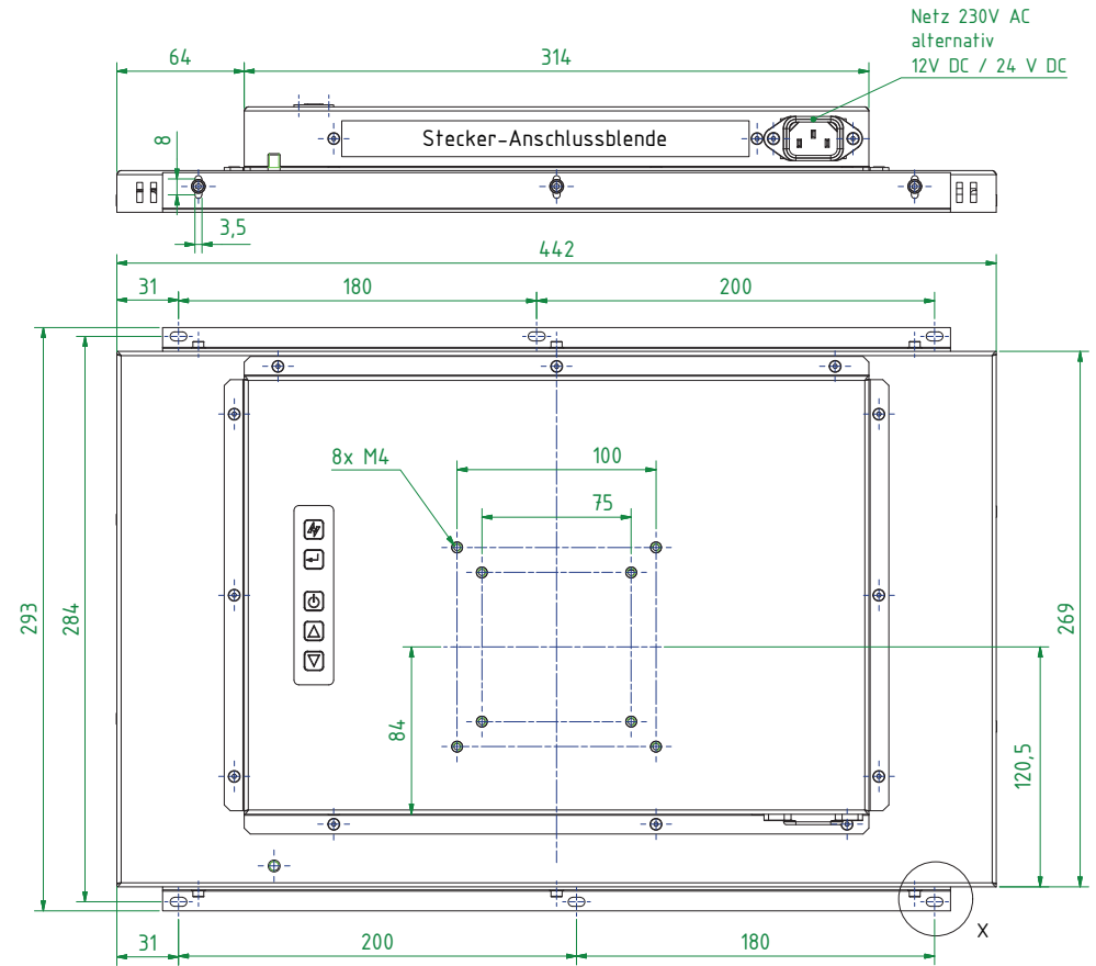
Rückansicht
