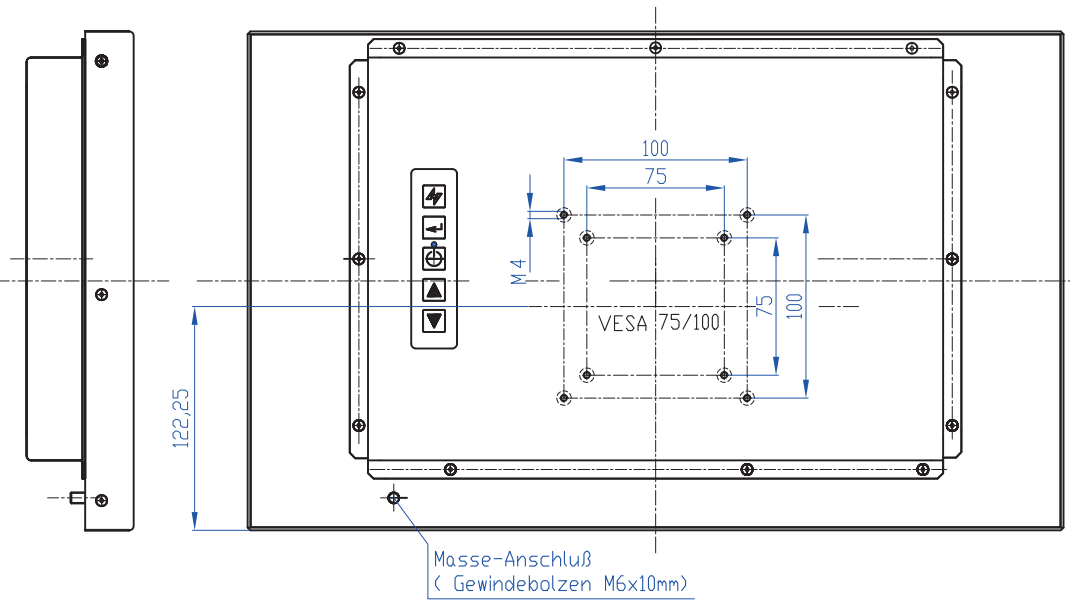
RÜCKANSICHT
