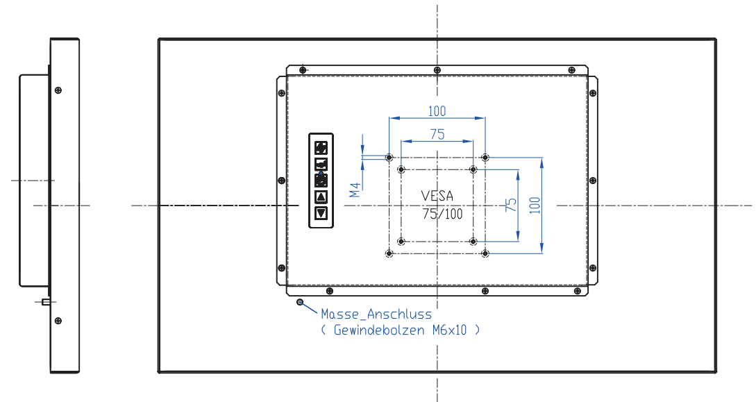
RÜCKANSICHT
