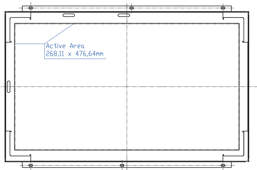
FRONTANSICHT
