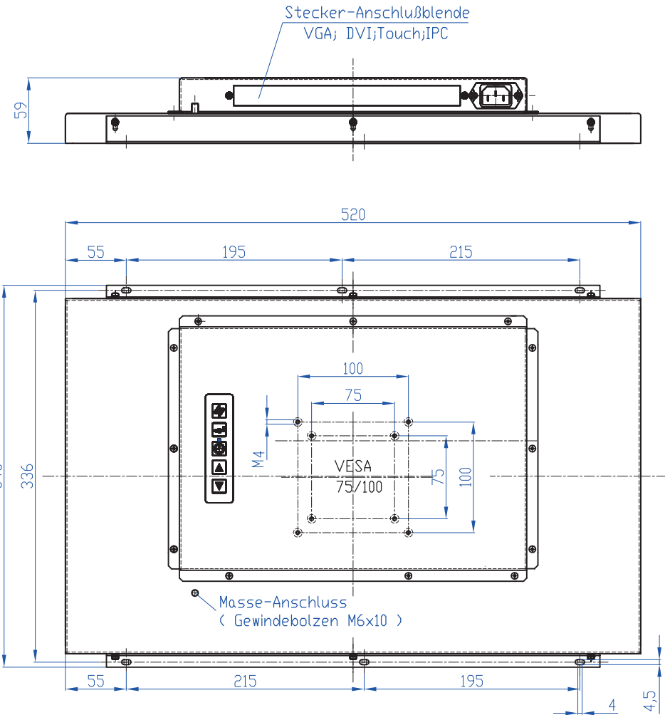
RÜCKANSICHT
