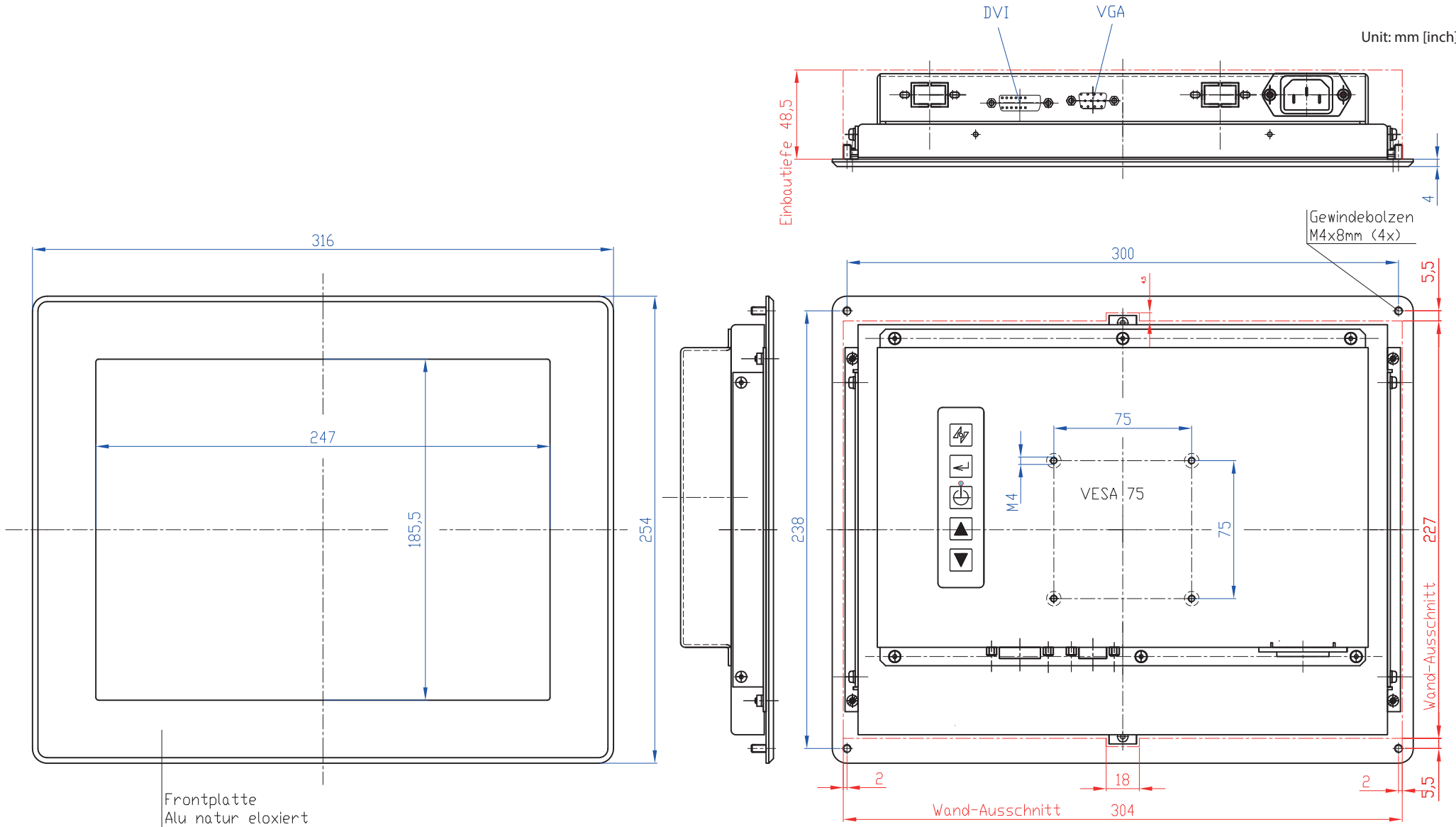
RÜCKANSICHT
